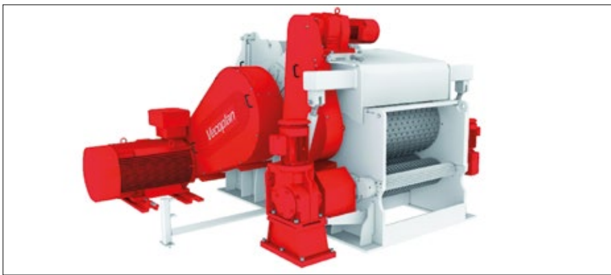
Барabanная рубительная машина Vecorplan для переработки древесины
